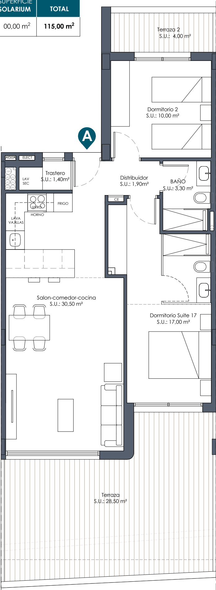
PLANTA PRIMERA
