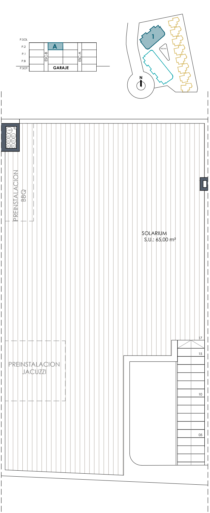
PLANTA ATICO
