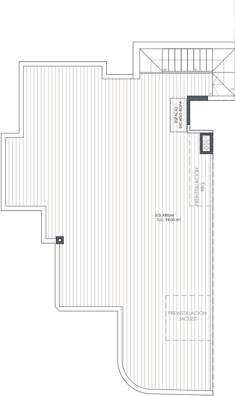
PLANTA SOLARIUM
